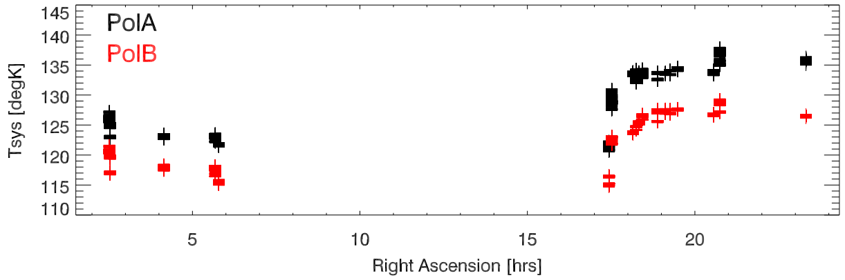
220209 Tsys vs RA (using 1sec offSrc samples). freqBand:9168
