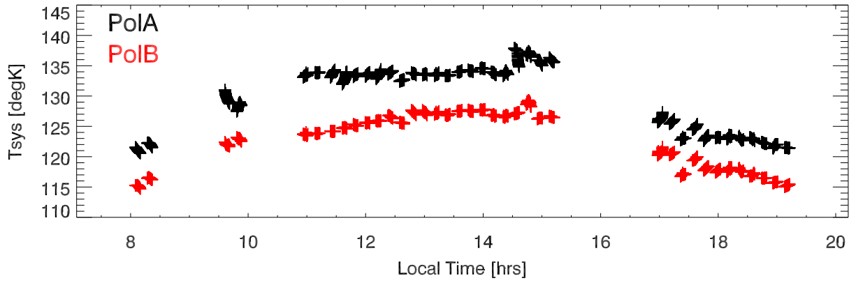
220209 Tsys vs Local Time (using 1sec offSrc samples). freqBand:9168
